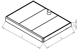
EMP.3545-6D
