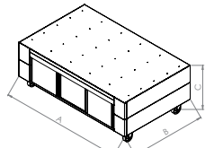
EMP.4060-3G-M
